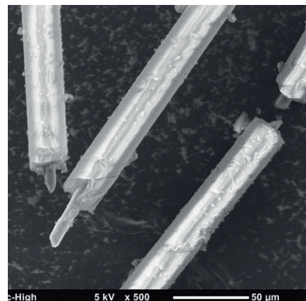
Рис. 2. Ферромагнитный микропровод
